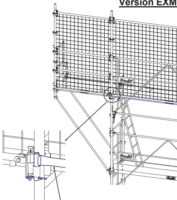
Longeron de 3m avec goupille bêta pour fixation filet (50230 )
