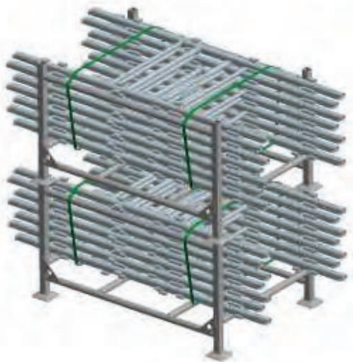
Exemple de conditionnement: Cadres F3000 (50030) rangés et cerclés dans des racks (23101)
